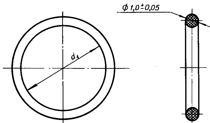
Размеры, мм
